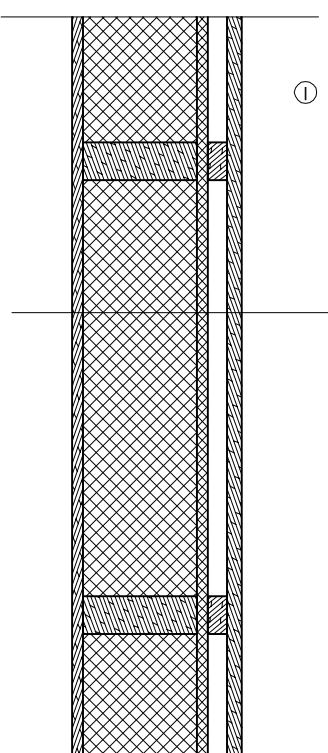
VERANDA VÄLISSEINA HORISONTAALLÕIGE
