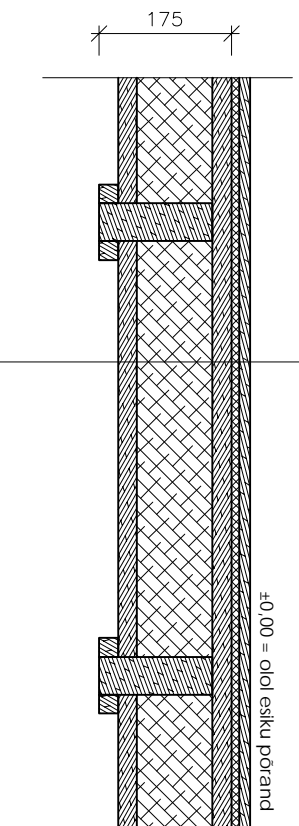
SAALI PÕRANDA LÕIGE
