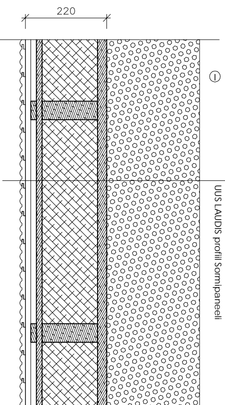
SAALI VAHELAE LÕIGE
