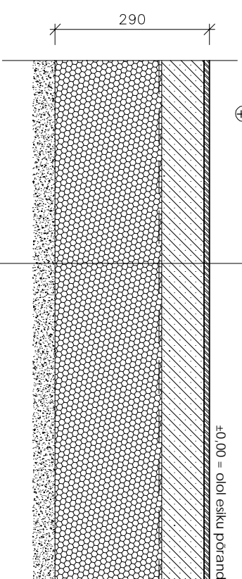
VERANDA PÕRANDA LÕIGE
