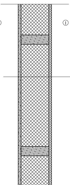
VERANDA LAE LÕIGE
